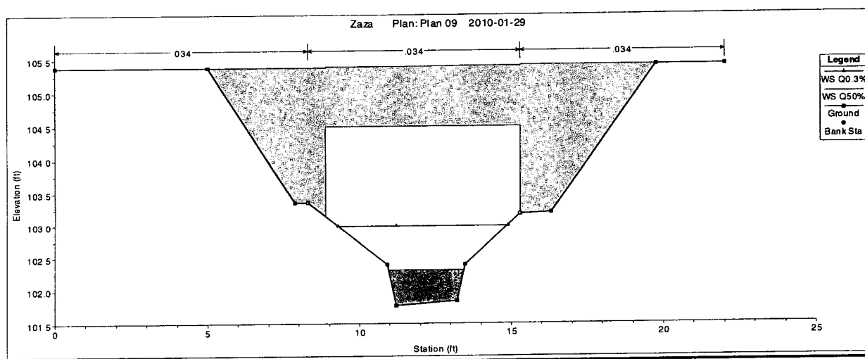
Rys.3. Przekrój poprzeczny koryta rzeki poniżej projektowanego mostu.
